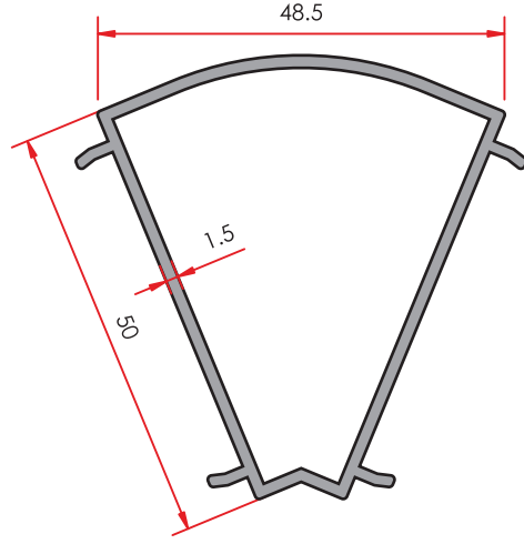
135 ° CORNER TURNING 135 ° KÖŞE DÖNÜŞ
