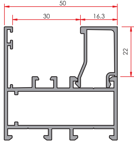
STRIP ÇITA
